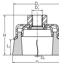
Cardas vaso
