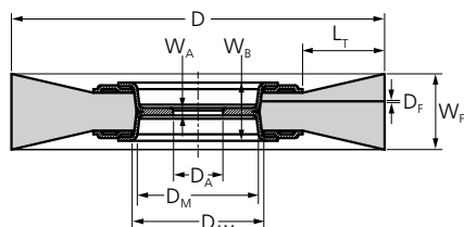
Cardas redondas
