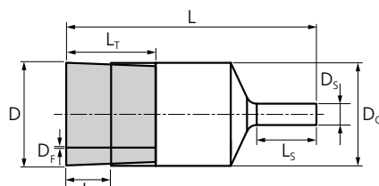
Cardas brocha
