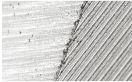
Nicht verrundete Schneidkante.
