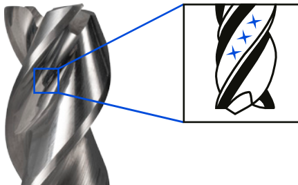
Polierte Spanräume für eine optimale Spankontrolle.
